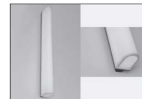
Applique Tennessee WL 96 Structure en aluminium, laiton et diffusant papier blanc. Finition en bronze. Eclairage blanc chaud 2200K à LED, 18W, 900Lumens. Convertisseur 24V à déporter. Poids : 4kg. Dimensions : 96,2x13,8x7,2cm. Conformité CE: Class III.
